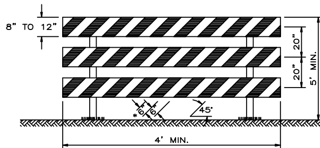
TYPE III BARRICADE
